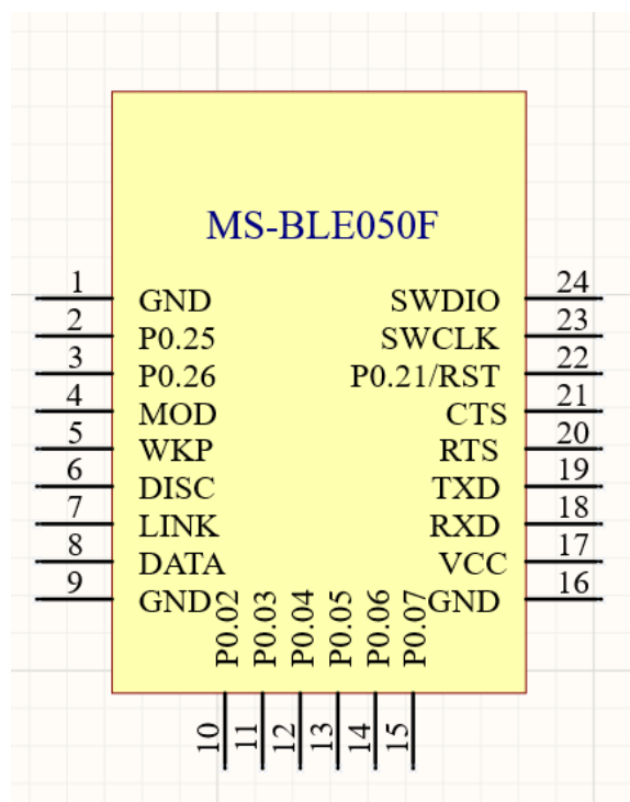
图 2 蓝牙模块引脚图
