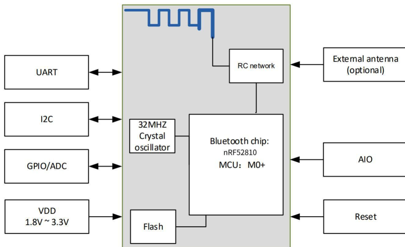
图1 MS-BLE050F 框架图
