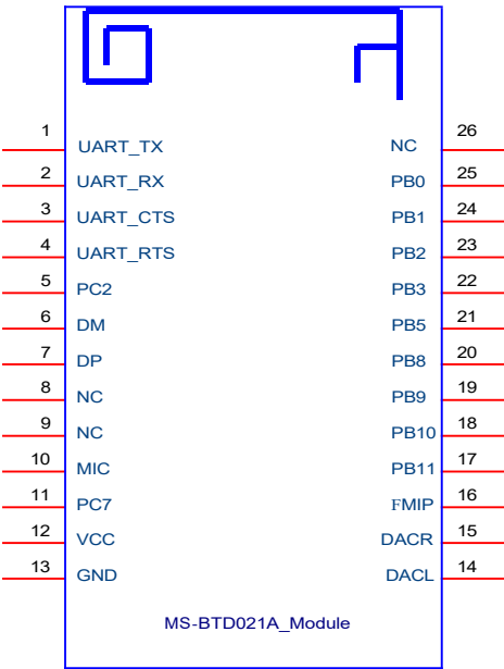
图 2 MS-BTD021A引脚图
