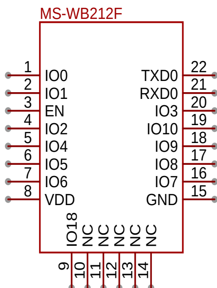
图 2 蓝牙模块引脚图
