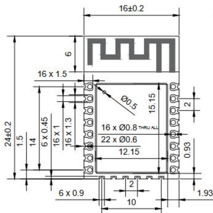
图 4 模块尺寸图
