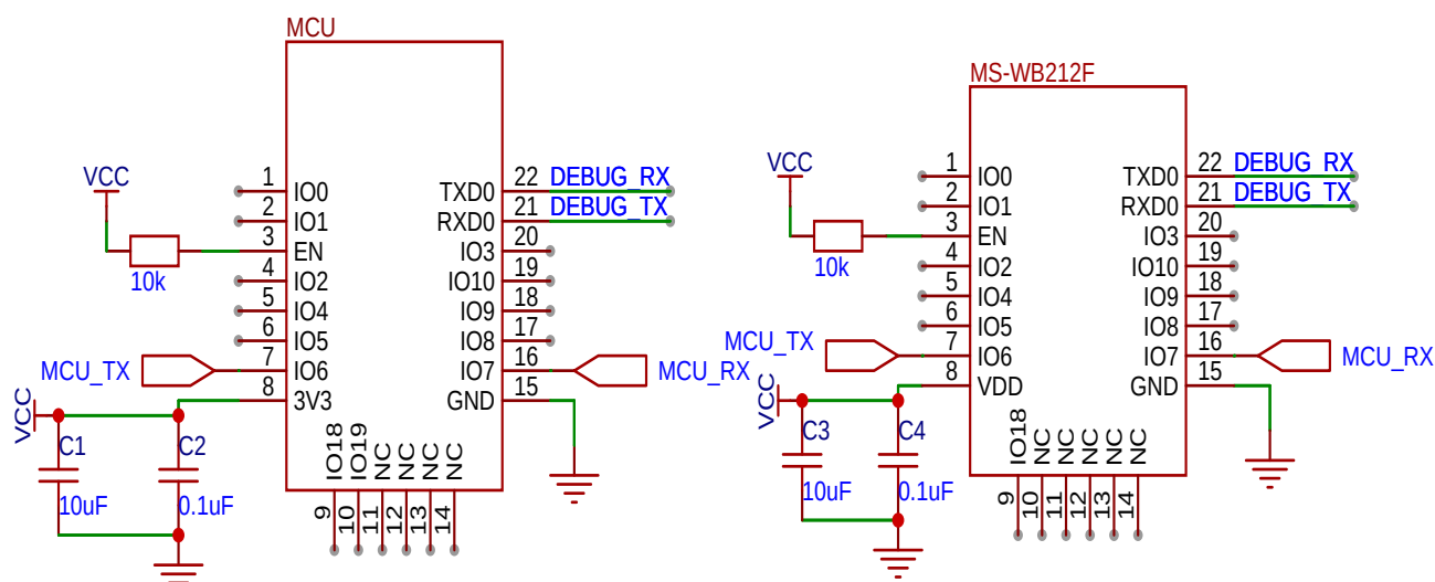
图 3 参考原理图
